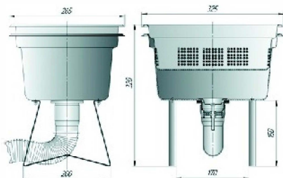
Мезгосборник К-200.25.000 СБ (К-150, К-200, К-300 )
